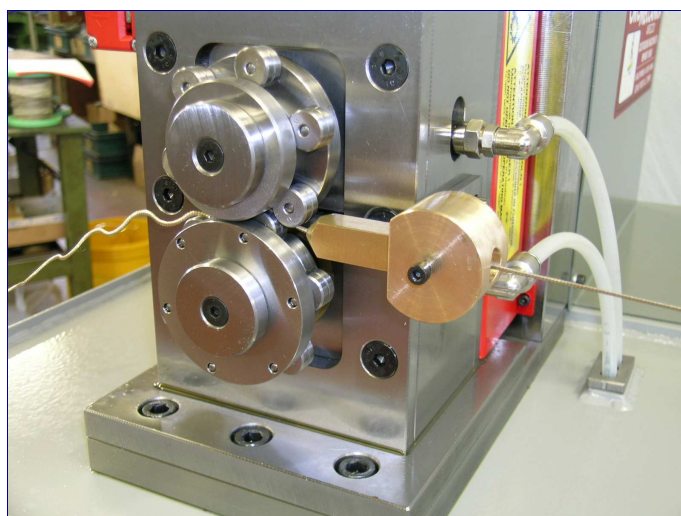
DISPOSITIVO SPECIFICO PER CATENA OMEGA
